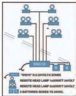
Central Control Unit รุ่น SN, SN LED
