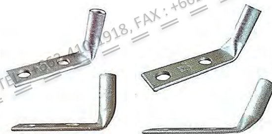
หางปลาแรงสูงชนิดรูคู่ 90°, 135°
