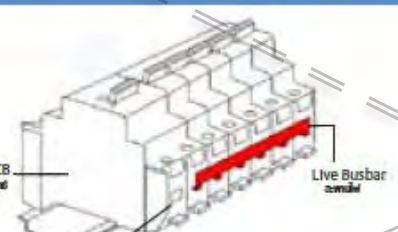
Fixing Busbar การติดตั้งคานาไฟ
